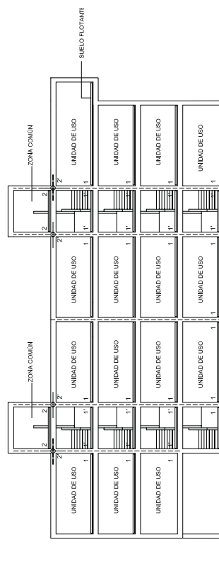
Disposición de suelos flotantes para limitar la transmisión de ruido de impactos entre recintos colindantes horizontalmente (1-1') y entre recintos con una arista horizontal común (2-2'). Figura 3.4. Esquema de sección vertical. Disposición de los suelos flotantes
